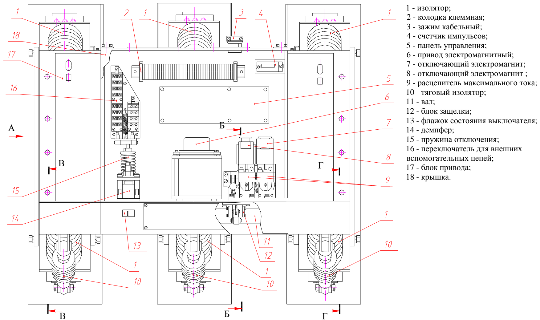
Рисунок В.2 Выключатель ВМС-35 УЗ
