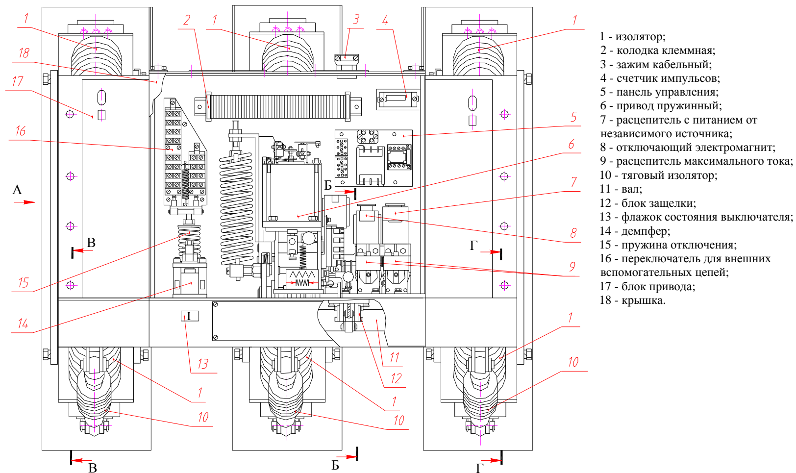
Рисунок В.1 Выключатель ВПС-35 УЗ
